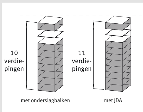
geringere constructiehoogte met JORDAHL® ponswapening JDA
